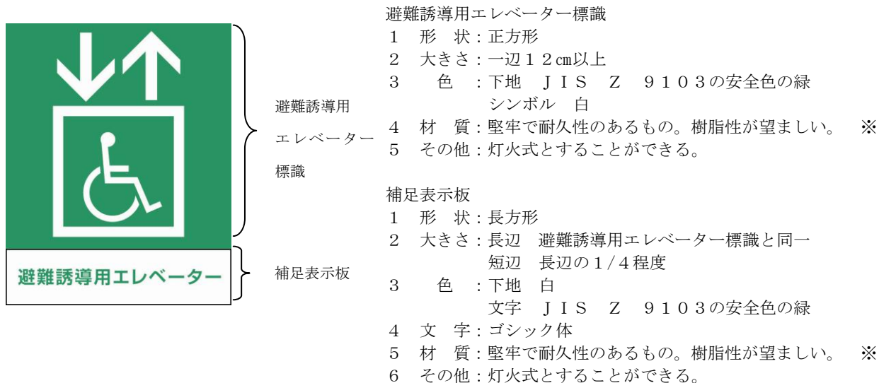
図1 避難誘導用エレベーター標識及び補足表示板
