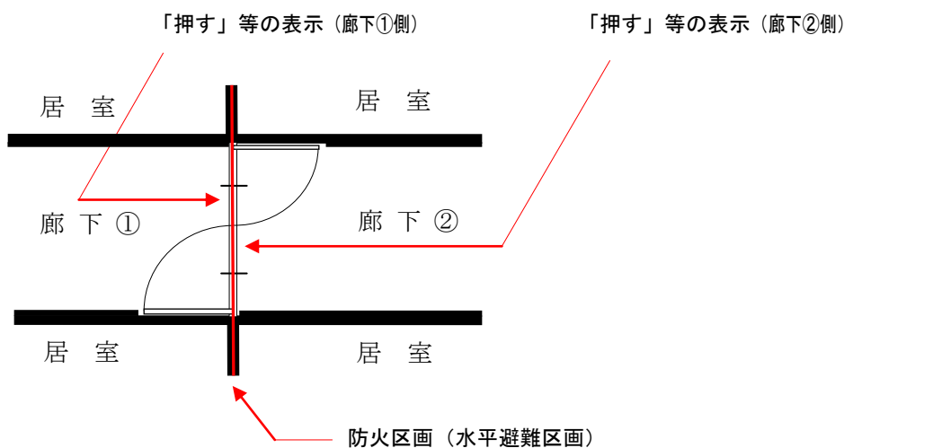
図7 水平避難区画の相互間に設ける防火設備（くぐり戸無し）の例
